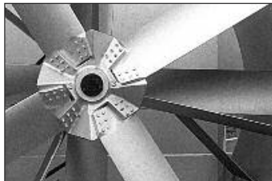
Vane-Axial Fan
